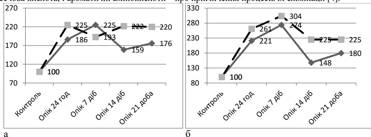
Рис. 1 Динаміка вмісту МСМ1 (А) і МСМ2 (Б) у сироватці крові тварин з хімічним опіком рогівки на тлі гіпотиреозу.
