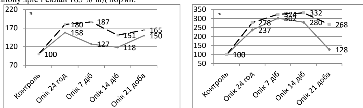
Рис. 2 Динаміка еритроцитарного (А) і лейкоцитарного (Б) індексів інтоксикації у кролів з хімічним опіком рогівки на тлі гіпотиреозу.
